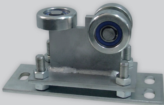
výškově nastavitelný vozík pro samonosné brány C profil 80×80
