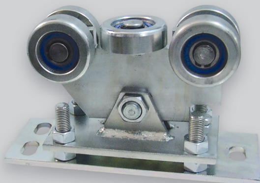
výškově nastavitelný náklonný vozík pro samonosné brány C profil 80×80
