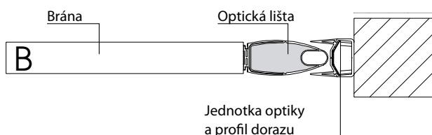
Obr. B - Krajní dorazový profil Nutné kódy 112000 + 112001 + 112002
