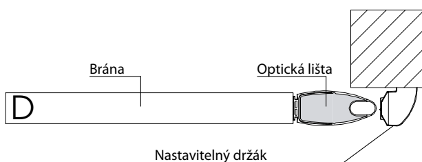
Obr. D - Nastavitelný nástěnný držák Nutné kódy 112000 + 112001 + 112003
