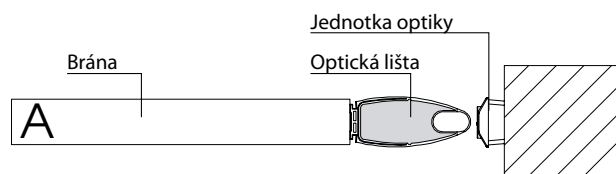
Obr. B - Krajní dorazový profil Nutné kódy 112000 + 112001 + 112002
